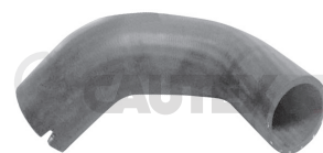
767110 Ø 56,00 mm radiator hose P 230- P 270- P 310- P 340- P 360- P 380- P 400- R 270- R 340- R 360- R 380- R 400-114 C/330-114 G/320-114 C/340-114 G/340-114 C/380-114 G/330-114 C/360- G oe: 1854058 -- 1380106
